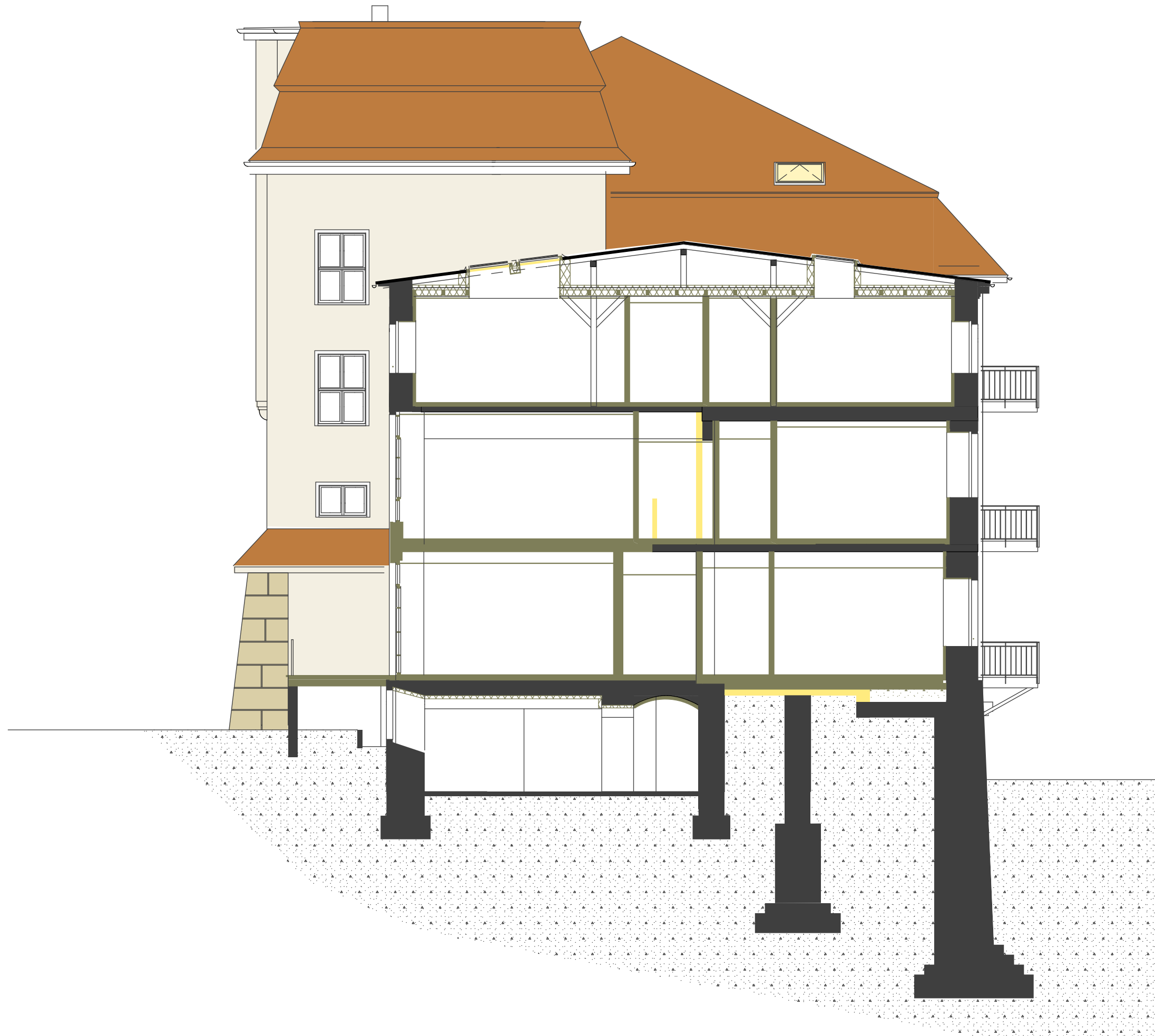
Ansicht Westen /Schnitt
